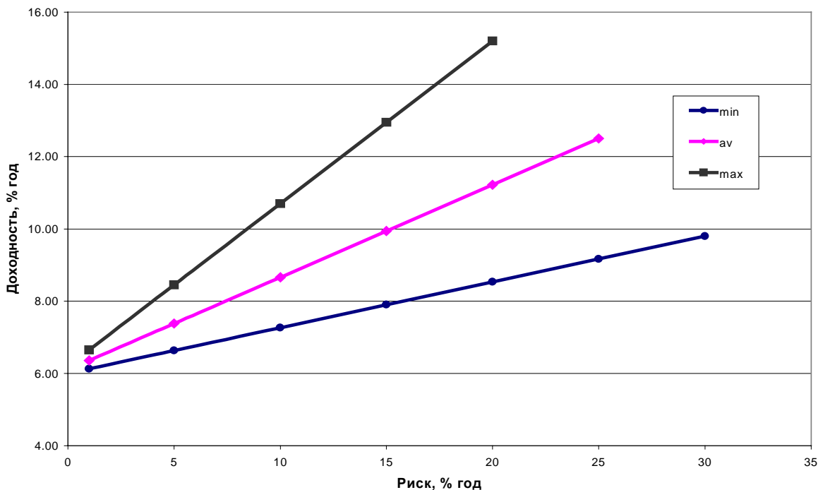
Рис. 9. Эффективная граница в виде полосы с линейными границами
