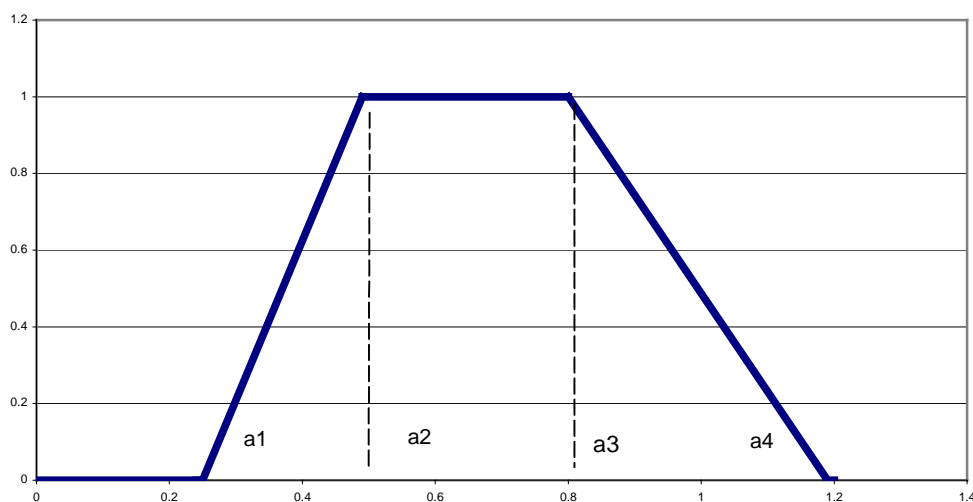
Рис. 4. Функция принадлежности трапецеидального числа
