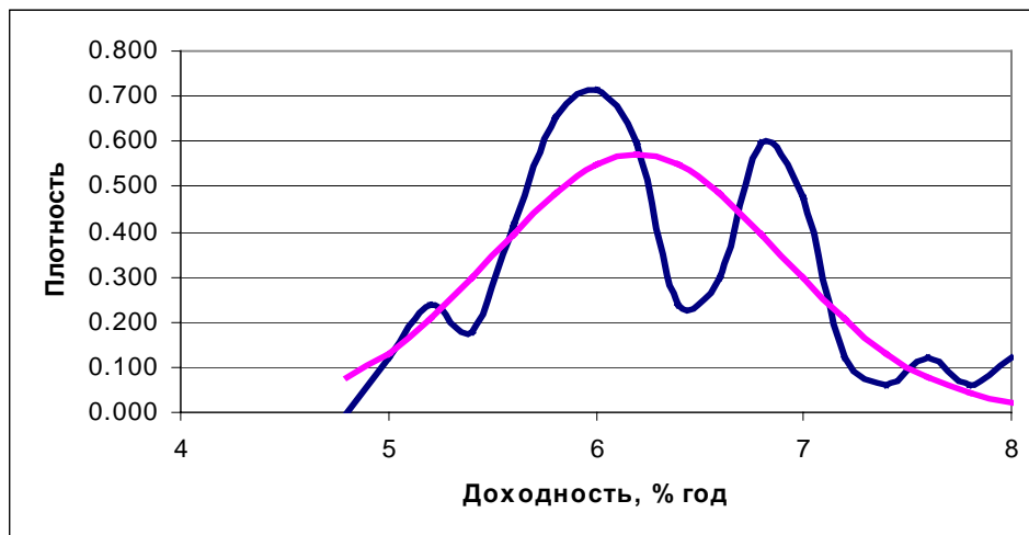
Рис. 8. Соотношение теоретической и экспериментальной плотностей распределения
